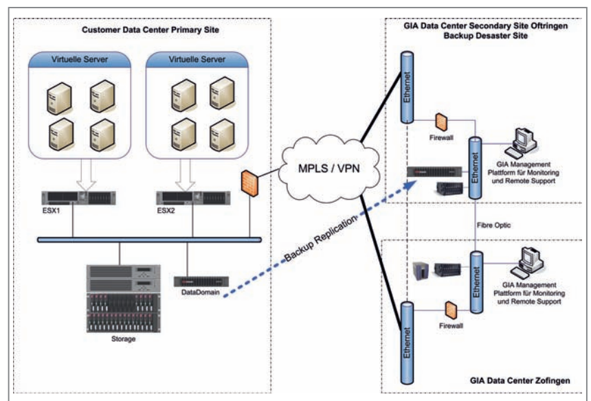
Replikation der Backup Daten in das Rechenzentrum von GIA.
